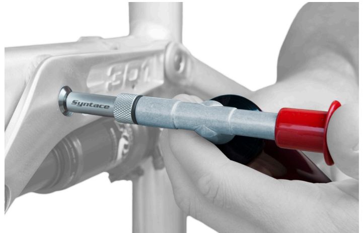
Anwendungsbeispiel ohne Aufsatzmundstück an einem Liteville-Rahmen 301 MK11-2
